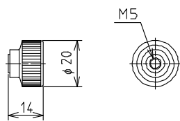
(3) Knob
